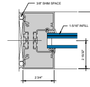
⑦ JAMB 6" = 1'-0"
