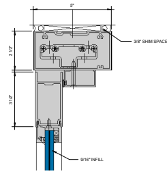
② COC HEADER OFFSET PIVOT 6" = 1'-0"
