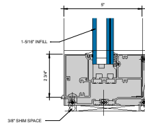
⑥ SILL 6" = 1'-0"
