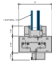
⑥ COC TRANSOM BAR OFFSET PIVOT 9" = 1'-0"
