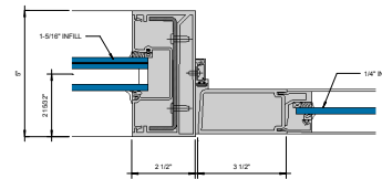
OPTIONAL DOOR JAMBS 5" x 1 1/2"
