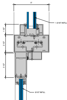
⑤ COC TRANSOM BAR OFFSET PIVOT 6" = 1'-0"
