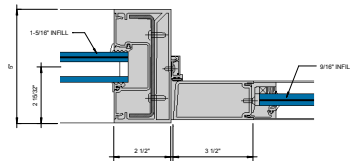
OPTIONAL DOOR JAMB 6" = 1'-0"
