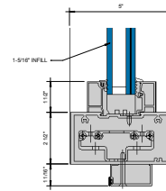
W/ LOC TRANSOM BAR OFFSET PIVOT 6" = 1'-0"
