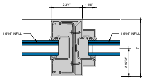
⑤ COC TRANSOM BAR OFFSET PIVOT 6" = 1'-0"
