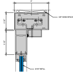
② COC HEADER OFFSET PIVOT Ø = 1'-0"
