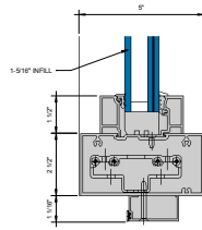
LOC TRANSOM BAR OFFSET PIVOT 6" = 1'-0"
