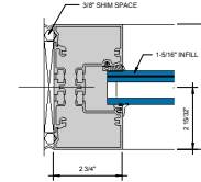
⑦ JAMB 6" = 1'-0"
