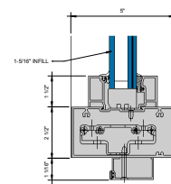
COC TRANSOM BAR BUTT HINGE 6" = 1'-0"
