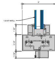
COC TRANSOM BAR OFFSET PIVOT 6" = 1'-0"
