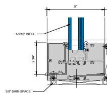
⑥ SILL 6" = 1'-0"
