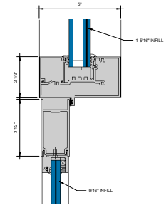
④ TRANSOM BAR Ø = 1'-0"
