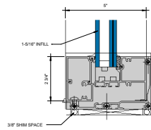
⑥ SILL 6" = 1'-0"
