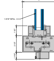
LOC TRANSOM BAR BUTT HINGE 6" = 1'-0"
