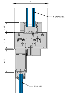
⑤ COC TRANSOM BAR OFFSET PIVOT 6" = 1'-0"
