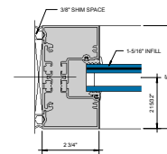
⑦ JAMB 6" = 1'-0"
