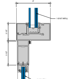
④ TRANSOM BAR 6" = 1'-0"
