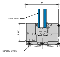
⑥ SILL 6" = 1'-0"
