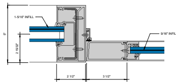
⑤ OPTIONAL DOOR JAMB 9" = 1'-0"
