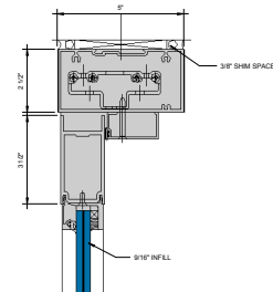
② COC HEADER OFFSET PIVOT 6" = 1'-0"
