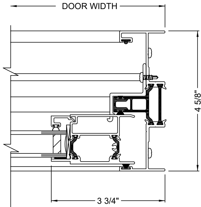
⑦ FIXED RIGHT JAMB
