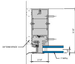
⑤ SGT JAMB - 1" INFILL 6" x 1'-0"
