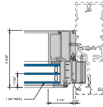
⑤ RIGHT JAMB PO. - 1-3/4" INFILL 6" = 1'-0"
