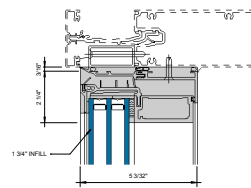
② HEAD COS. - 1-3/4" INFILL 6" = 1'-0"
