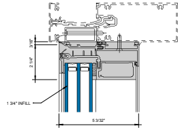
① HEAD PO. - 1-3/4" INFILL 6" = 1'-0"
