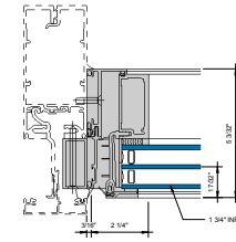
⑥ LEFT JAMB COS. - 1-3/4" INFILL 6" = 1'-0"
