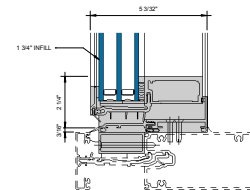
③ SILL POS. COS. - 1-3/4" INFILL 6" = 1'-0"
