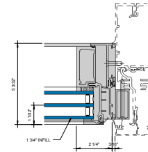
⑥ RIGHT JAMB PO - 1-3/4" INFILL 6" = 1'-0"
