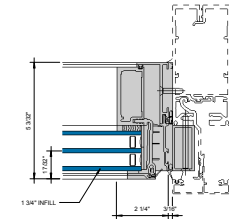
⑦ RIGHT JAMB COS. - 1-3/4" INFILL 6" = 1'-0"
