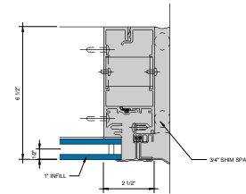
⑦ SGT JAMB - 1" INFILL 6" = 1'-0"
