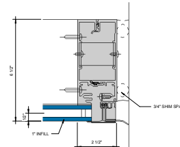
⑦ SGT JAMB - 1" INFILL 6" x 1'-0"
