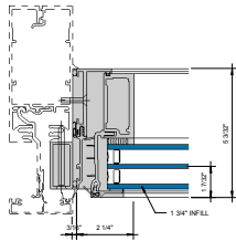
④ LEFT JAMB PO - 1-3/4" INFILL 6" = 1'-0"
